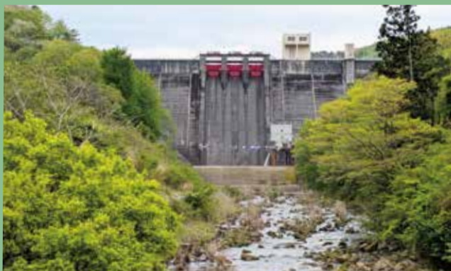
矢作川水系の巴川上流に昭和38年に築造された羽布ダム。
